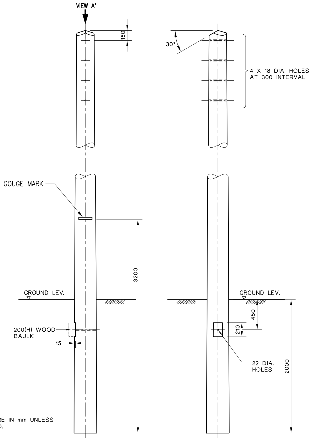
VIEW A'
